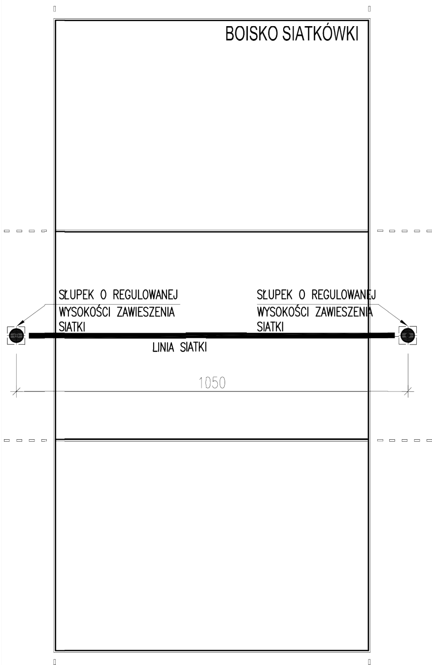
WIDOK 1:100
